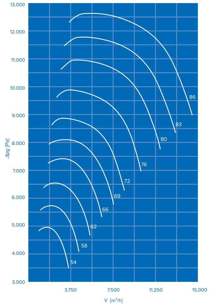
Kennlinie Ventilatorart PHD Drehzahl 2.900 1/min
